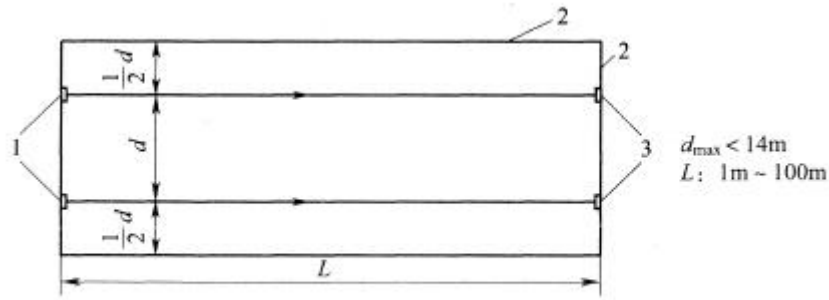
图7 线型光束感烟火灾探测器在相对两面墙壁上安装平面示意图
