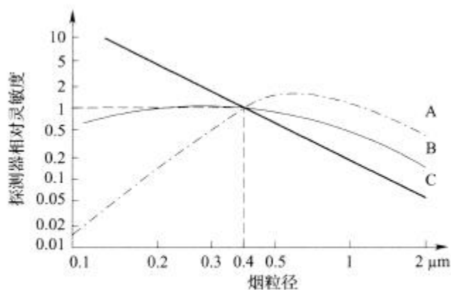
图 2 感烟火灾探测器对不同烟粒径的响应
