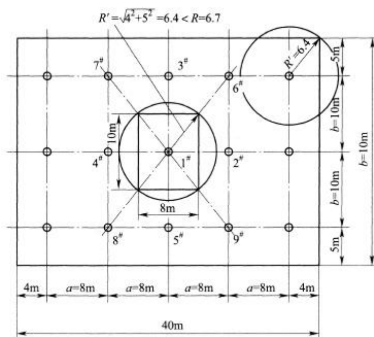
图 4 探测器布置示例
