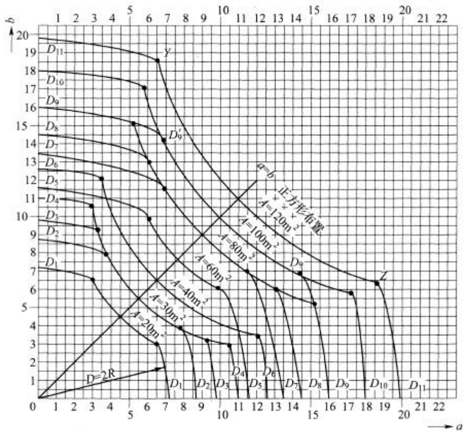
图 E 探测器安装间距的极限曲线
