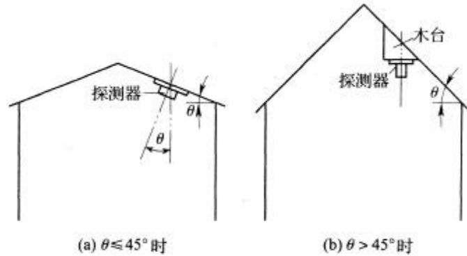
图 6 探测器的安装角度
